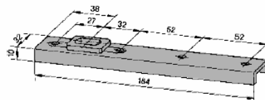
Ref. 8021 brazo soporte inferior para 100kg
