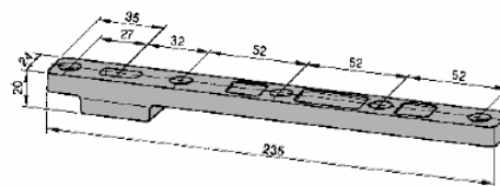
Ref. 7421 brazo soporte inferior para 300kg
