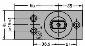
Ref. 7475AX punto de giro inferior hasta 300kg
